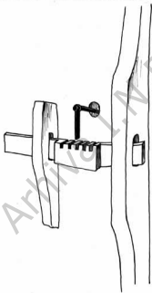
BIS. DE LEMN S TA VOEVOZI DIN BEREASA JUD. VASLUI - ZĂVÔRUL DE LEMN AL UȘEI
