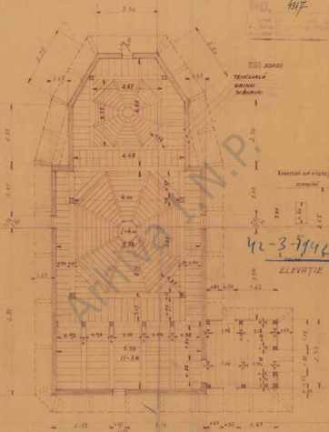
BIS ST IV VOLVOZI - BEREASA - JUD VASLUI - SCHIȚA DE RELEVIEU - SCARA OM02 = 1M.
