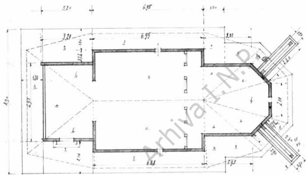
PLANUL FERTELUI LUCRĂRII DE CONSOLIDARE BIS. DE LEMN DIN COMUNA DRĂGUSENI DE SUS - JUDEȚUL DOROHOI SCARA 1:50-1 METRU
