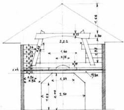
SECȚIE A-B
