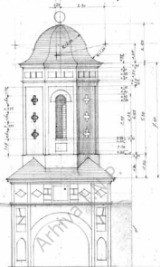
ELEVATIE
