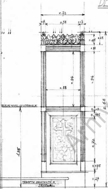
DETALIU MARIME DE EXECUTIE
