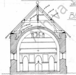
SECTIE TRANSVERSALA CU PROIECT PENTRU SARPANTA
